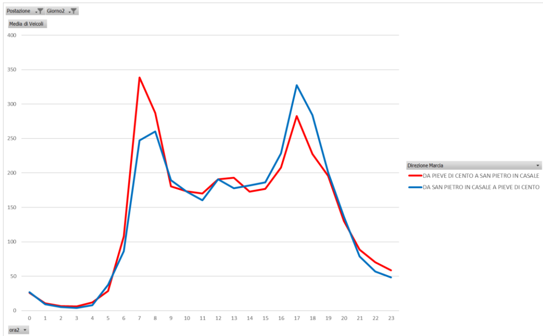
Fig. 2.26 Postazione 290 - Distribuzione dei flussi veicolari (Media mensile Lun-Ven )
