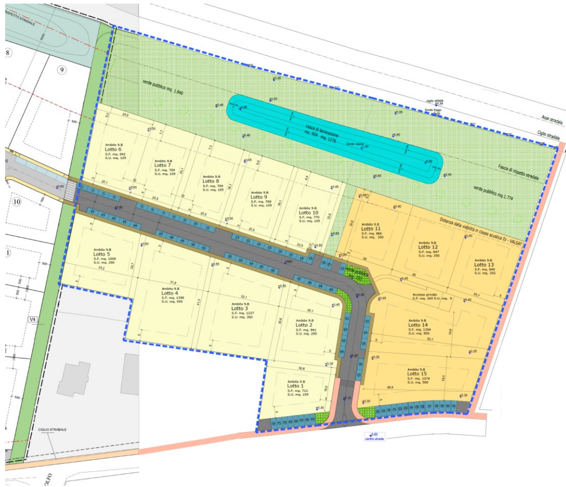
Fig. 2.10 – Planimetria progetto Sub-Ambito 9.B
