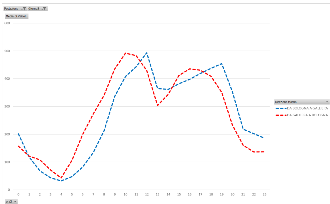
Fig. 2.31 Postazione 292 - Distribuzione dei flussi veicolari (Media mensile Sab-Dom )
