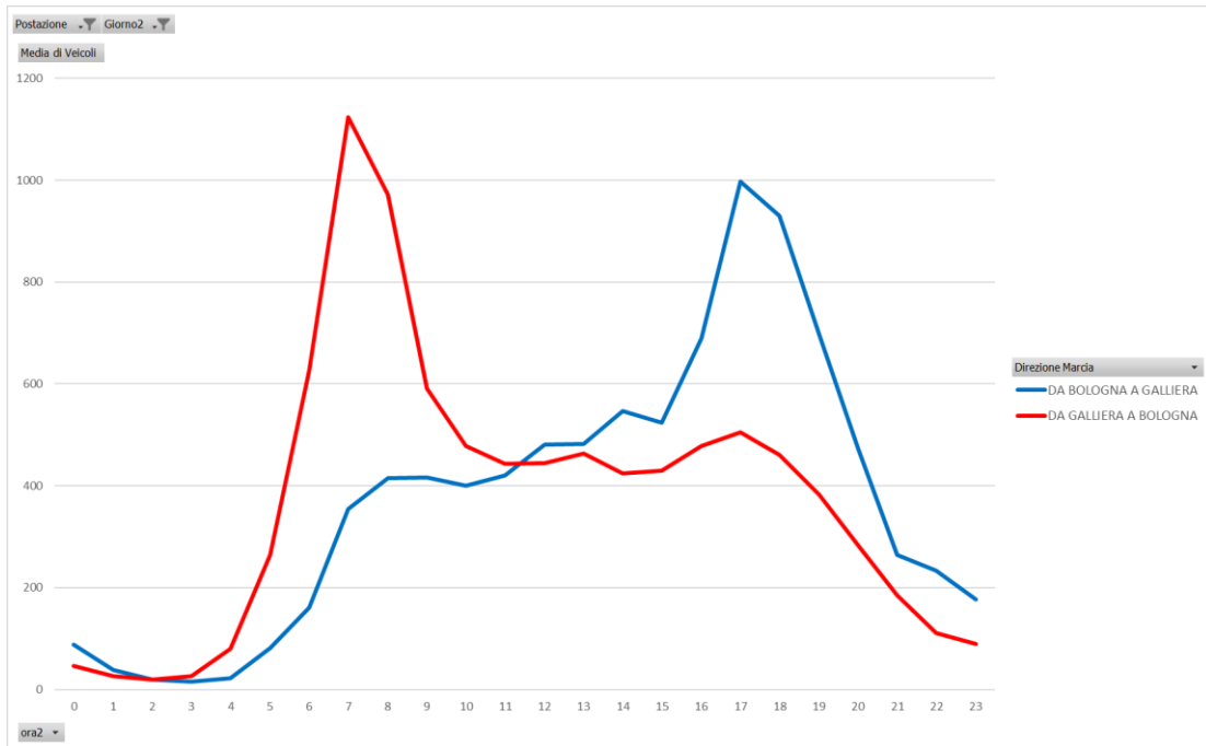
Fig. 2.28 Postazione 292 - Distribuzione dei flussi veicolari (Media mensile Lun-Ven )
