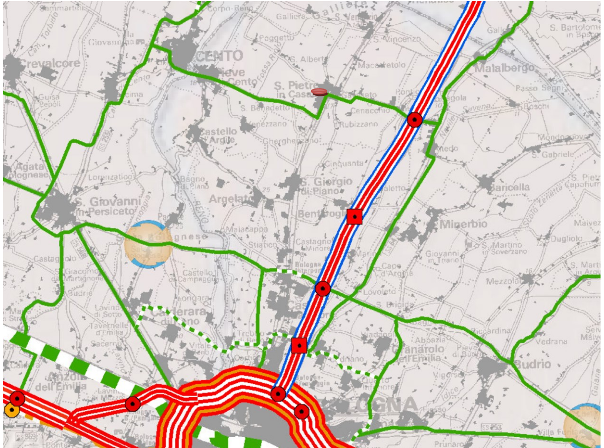
Fig. 2.23 – Classifica funzionale della rete stradale redatta dalla Regione Emilia Romagna (PRIT)
