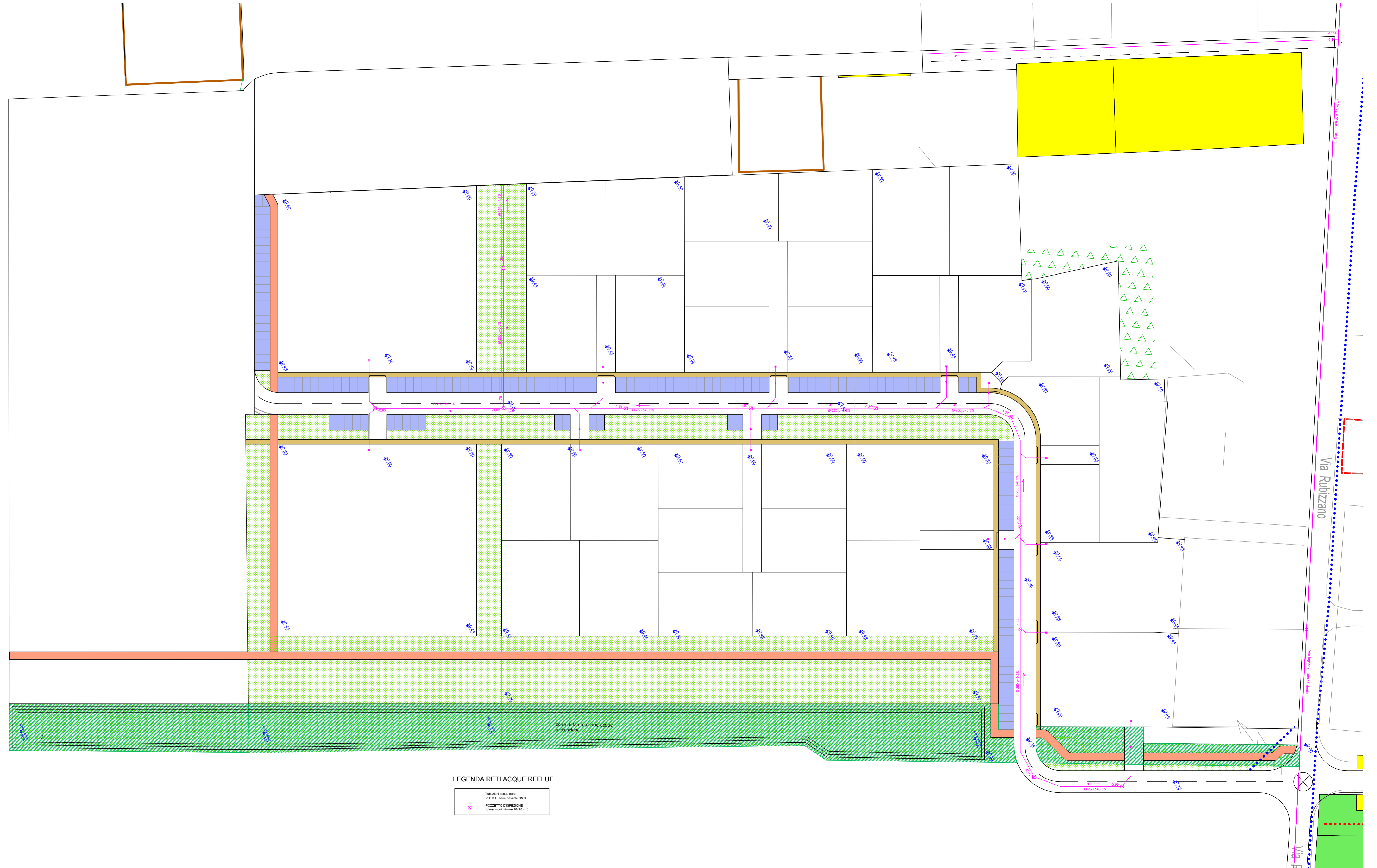
planimetria rete fognaria acque nere Sub Ambito 5.1 - scala 1:500
