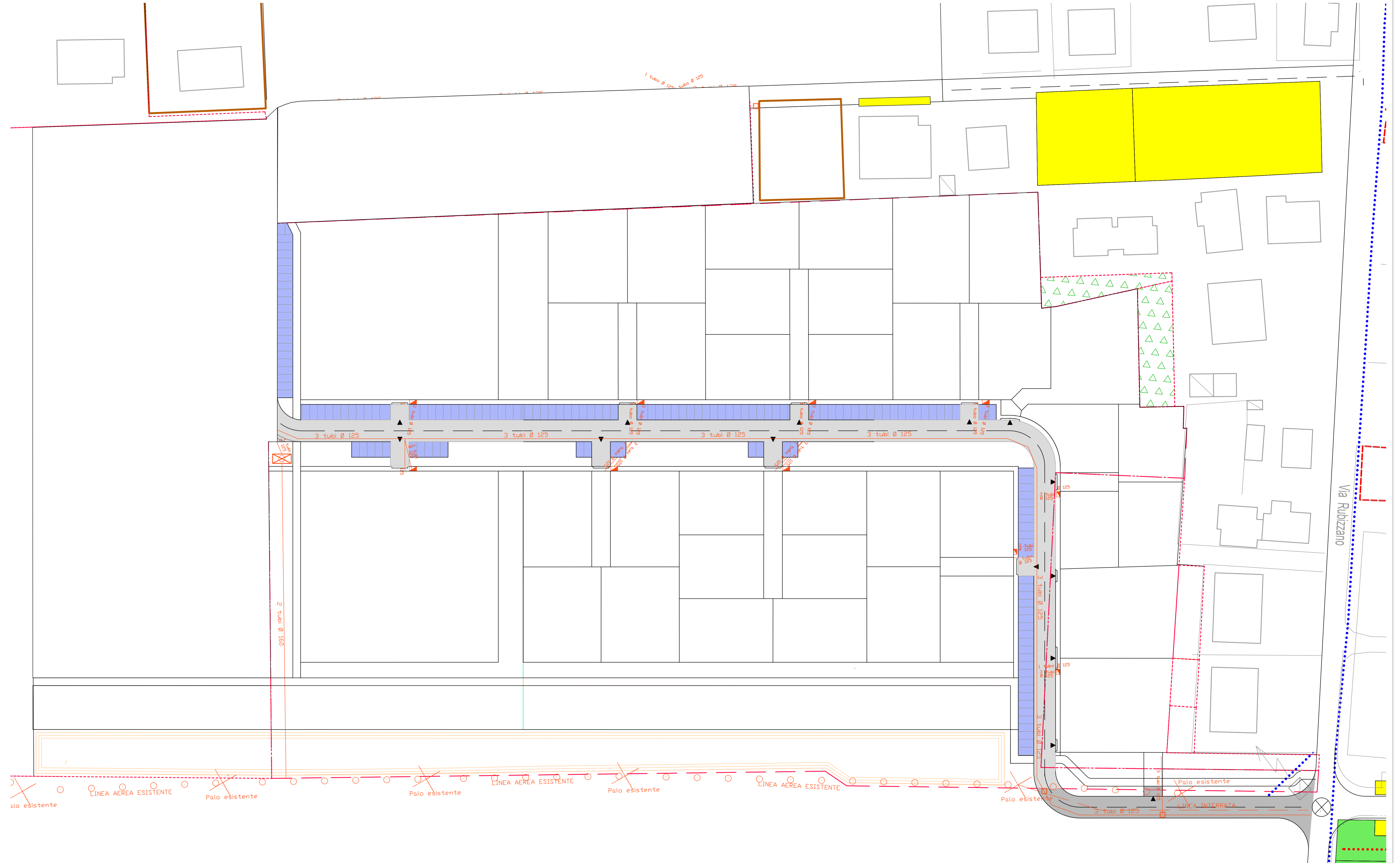
planimetria rete elettrica Sub Ambito 5.1 - scala 1:500
