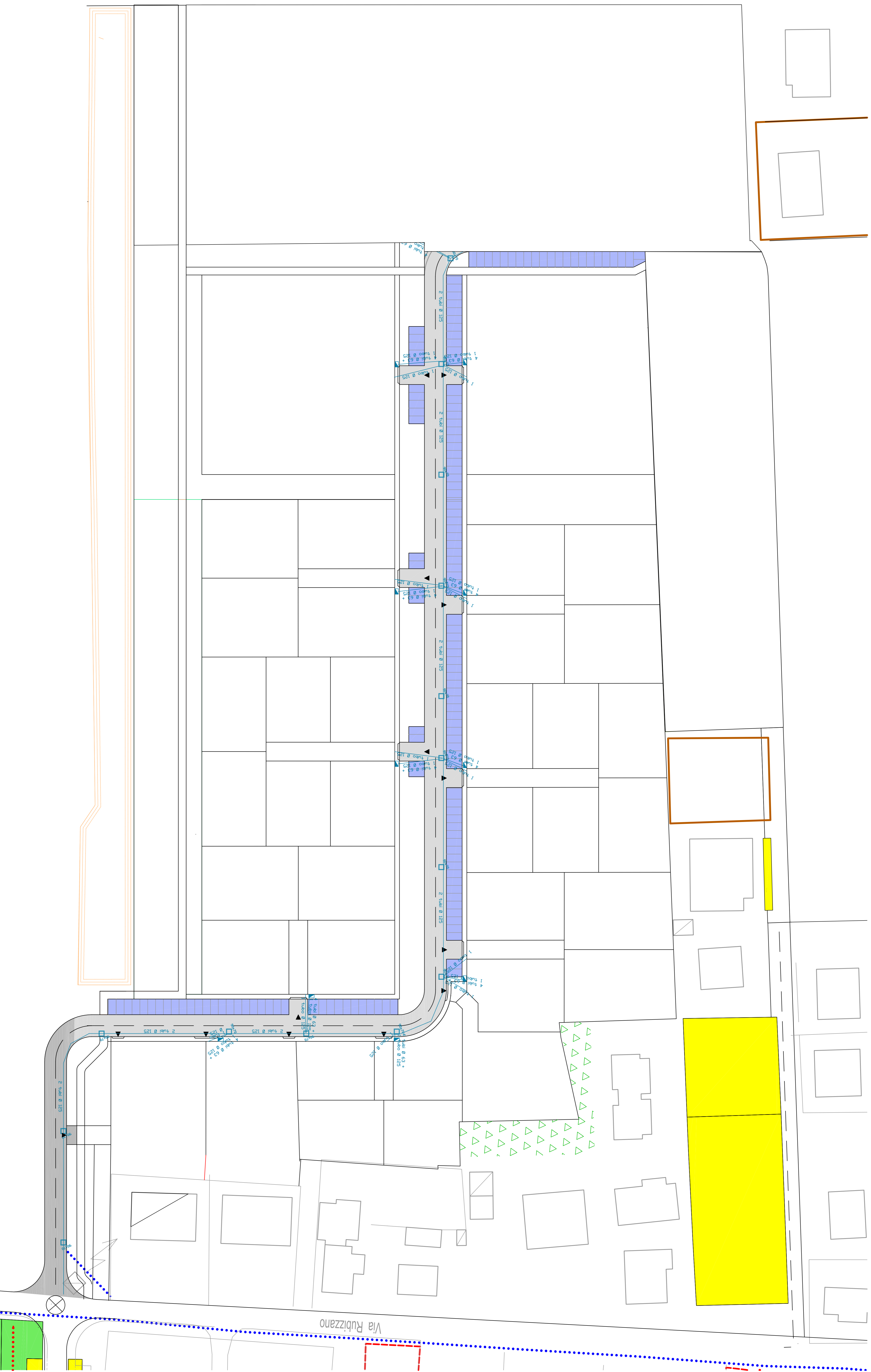
planimetria rete telefonica Sub Ambito 5.1 - scala 1:500
