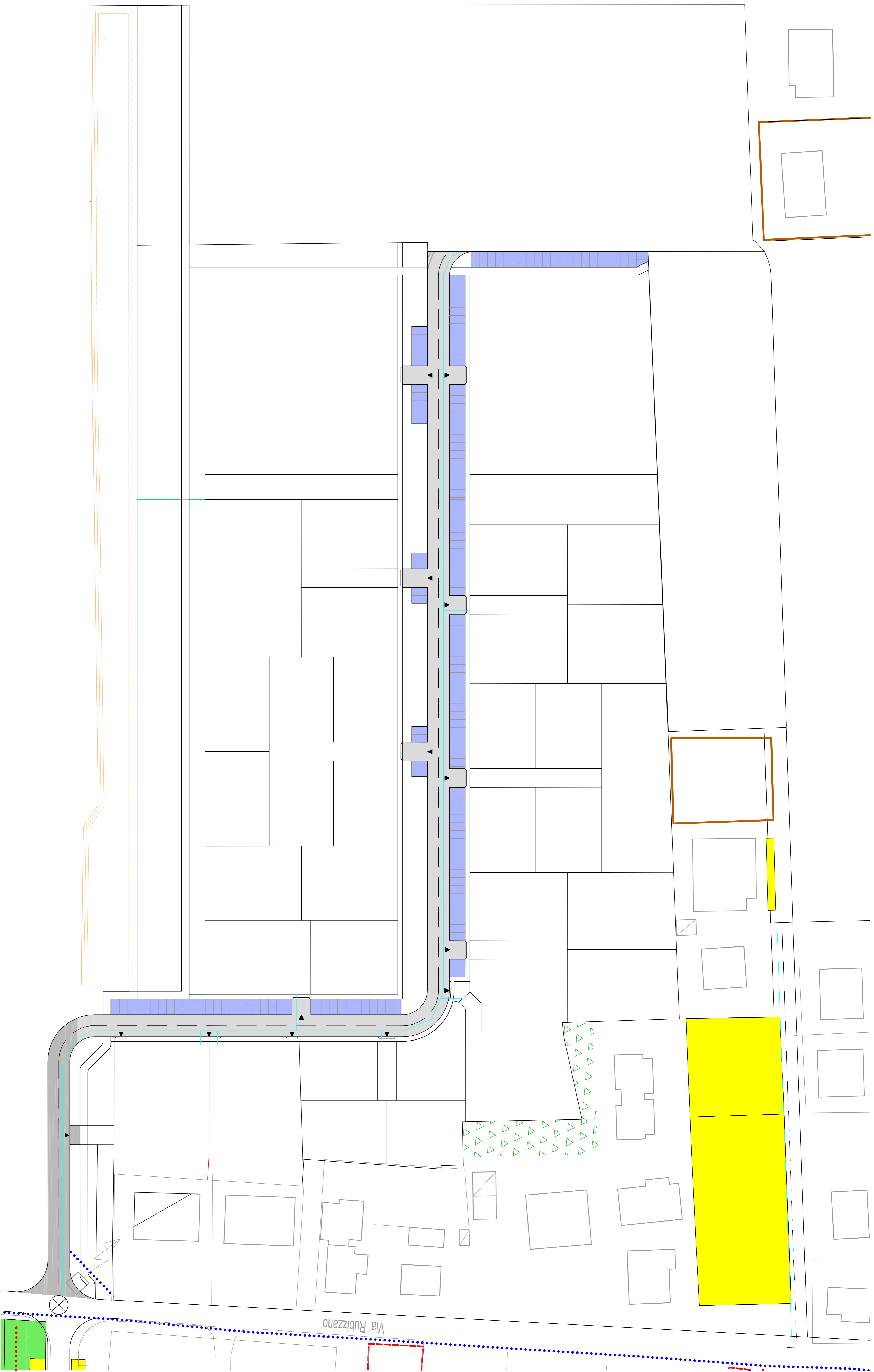
planimetria rete acqua Sub Ambito 5.1 - scala 1:500
