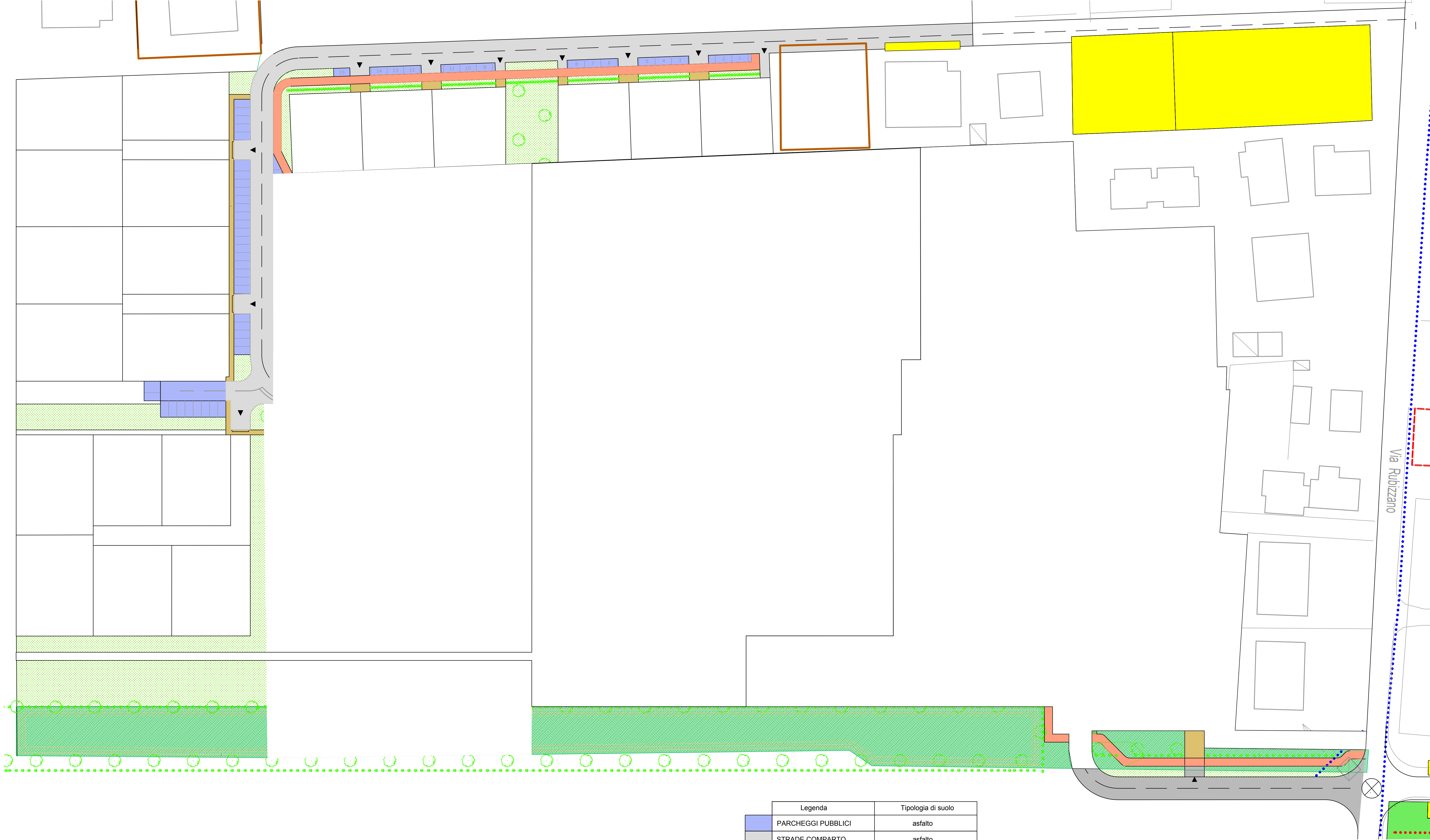
planimetria Sub Ambito 5.2 - scala 1:500
