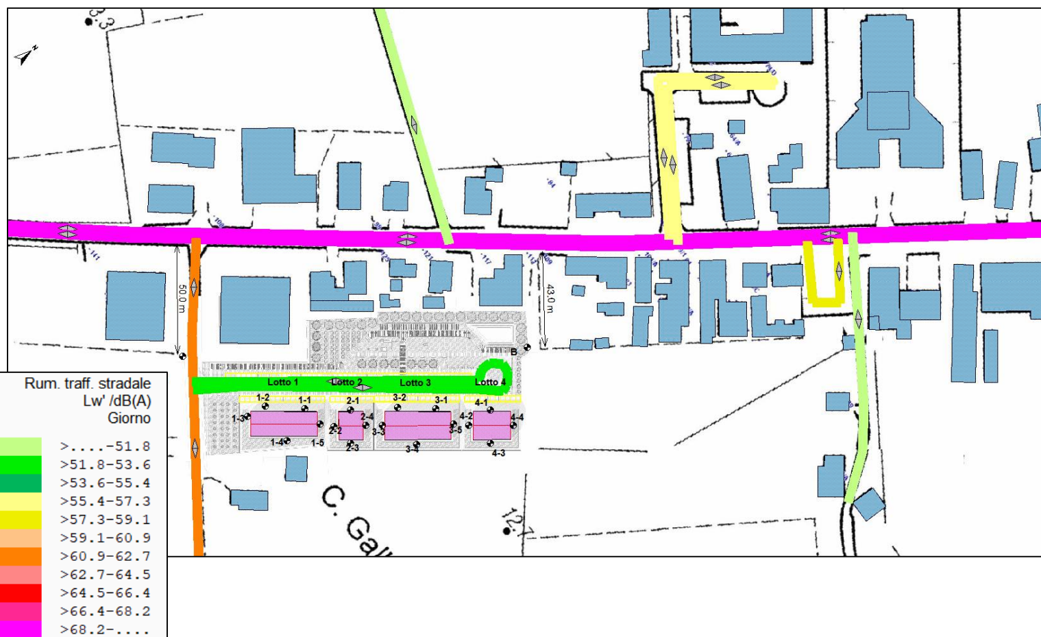
Immagine 11.2 – Livelli di potenza sonora allo stato di progetto delle arterie viarie sienite nel modello di calco IMMI vs. 2020
