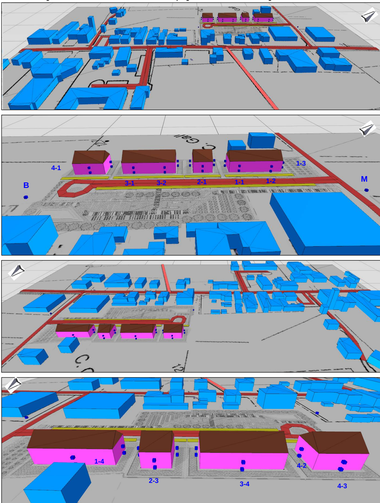
Immagine 11.1.2 – Modellazione tridimensionale di progetto e indicazione dei bersagli considerati
