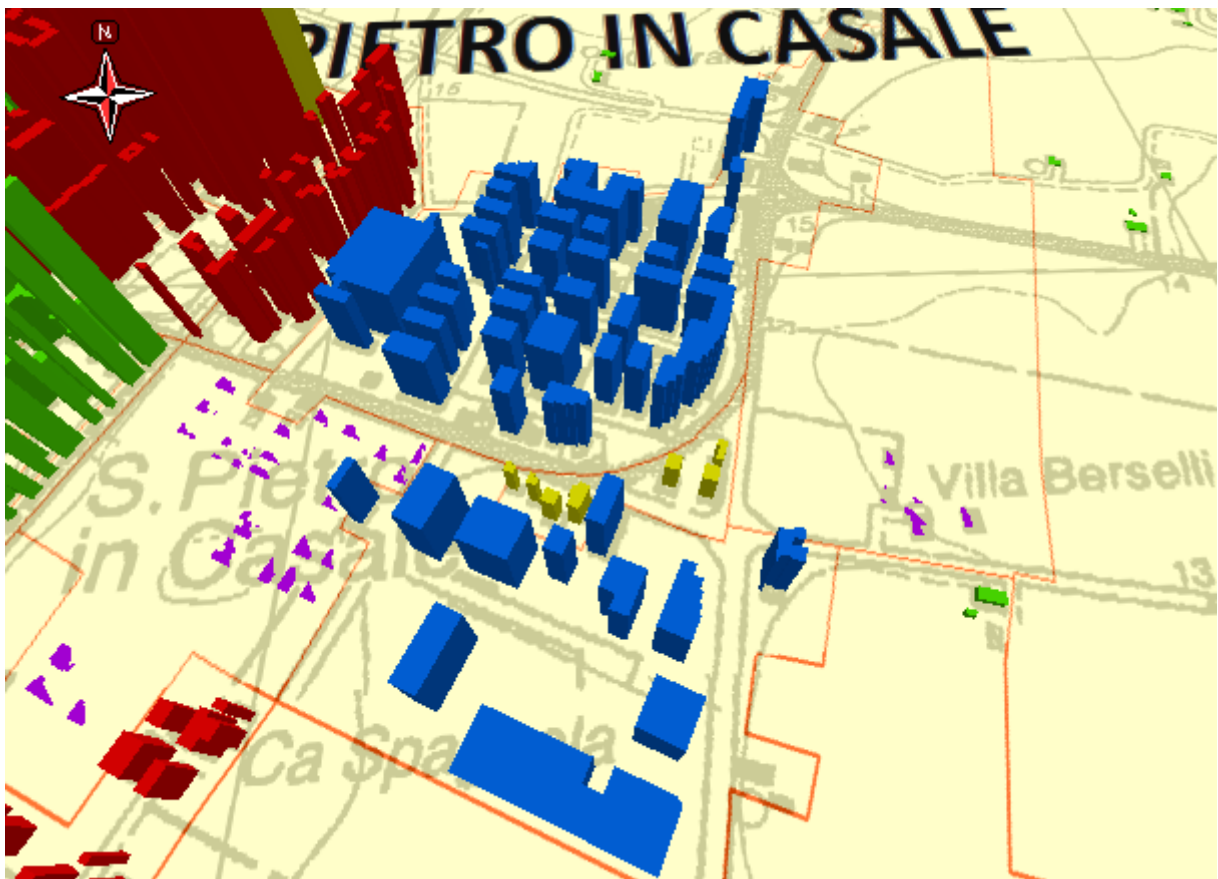
Figura 11: Particolare dei consumi elettrici industriali di SAN PIETRO IN CASALE. Anno 2008
