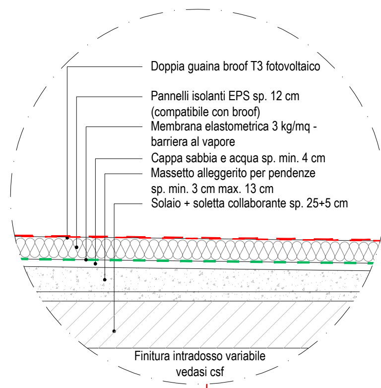
SOLAIO COPERTURA PIANA
