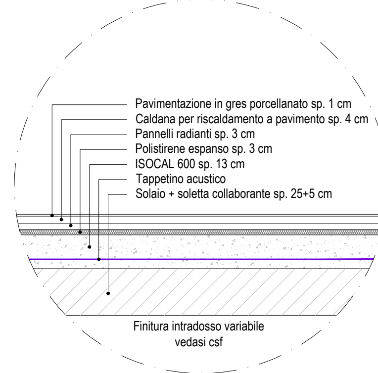
SOLAIO INTERPIANO ZONE RISCALDATE
