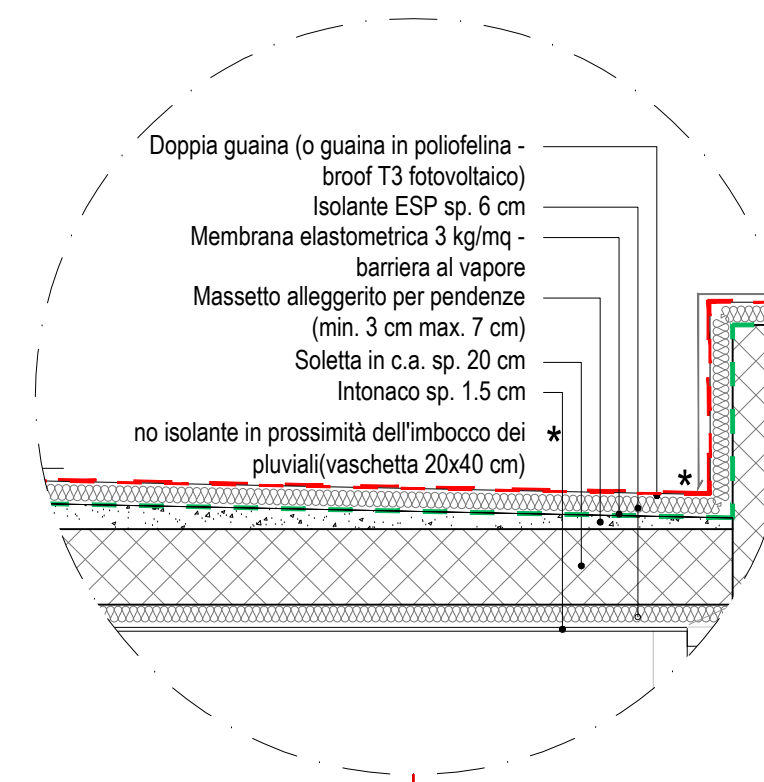
COPERTURA PENSILINA A SBALZO LATO SUD
