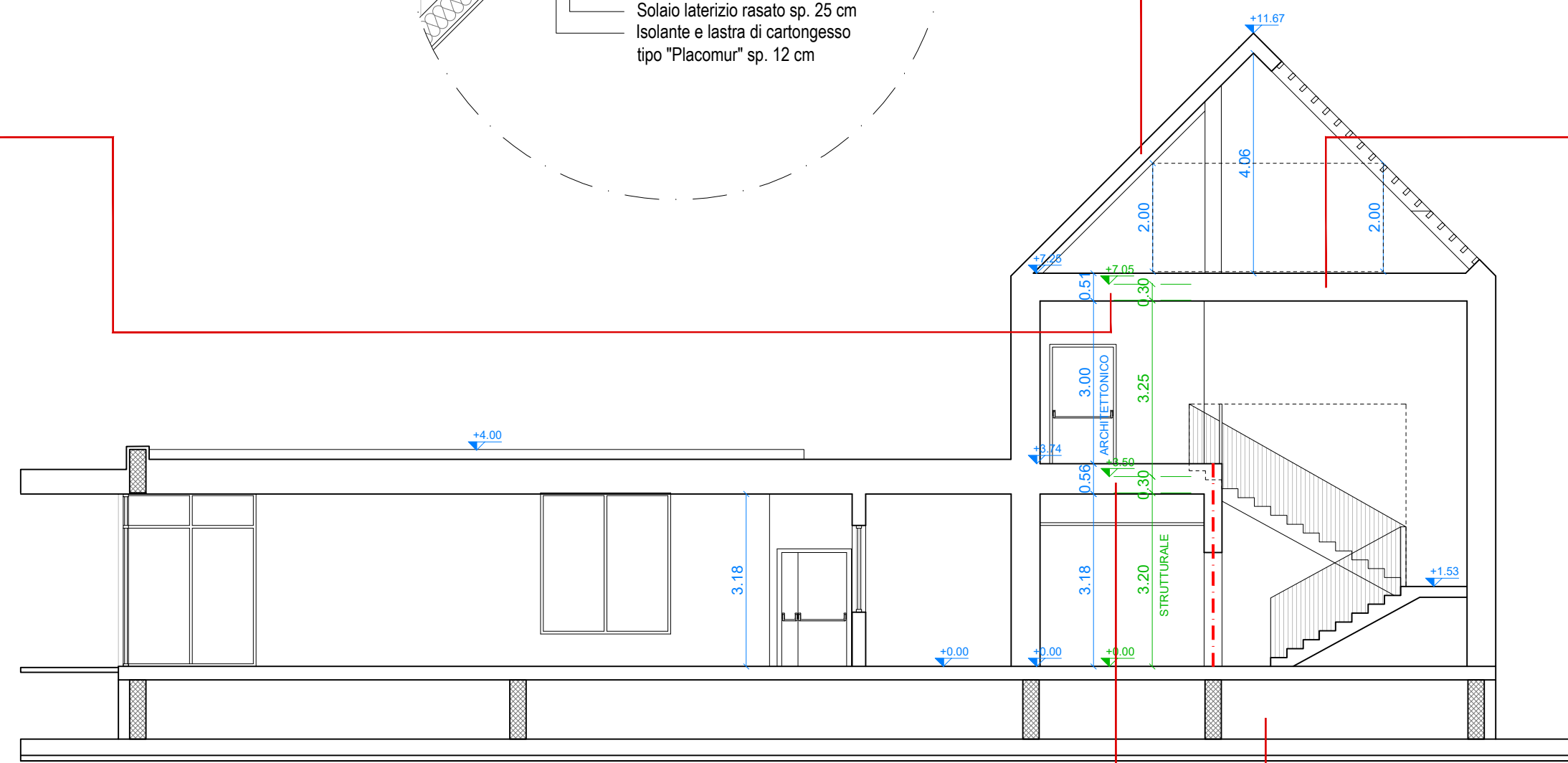
SEZIONE A-A'
