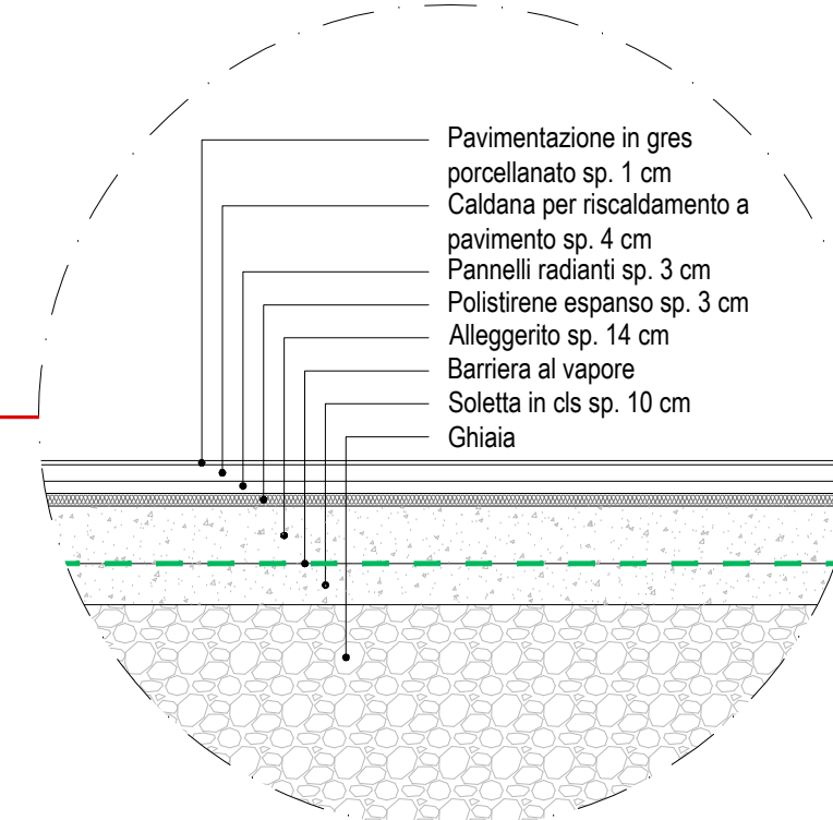
SOLAIO CONTROTERRA PIANO TERRA
