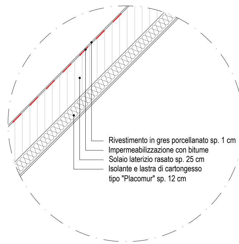
SOLAIO COPERTURA INCLINATA
