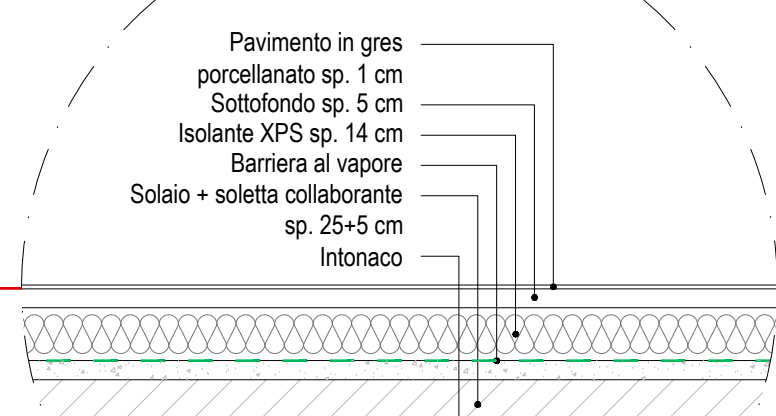
SOLAIO SOTTOTETTO PIAZZOLA POMPA DI CALORE
