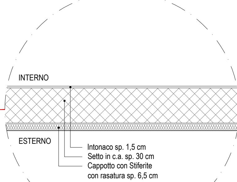
MURATURA ESTERNA TRASVERSALE sotto in c.a.
