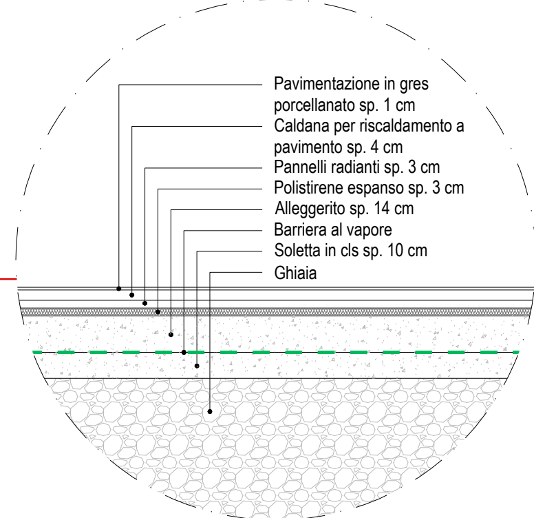
SOLAIO CONTROTERRA PIANO TERRA
