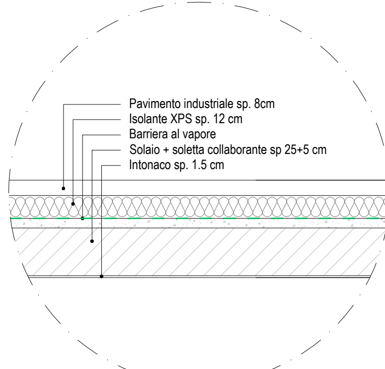
SOLAIO SOTTOTETTO
