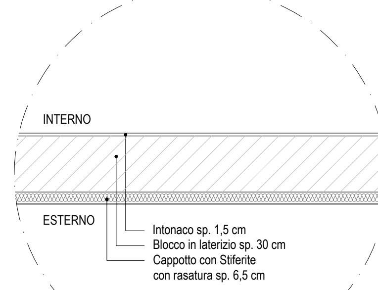
MURATURA ESTERNA TRASVERSALE laterizio
